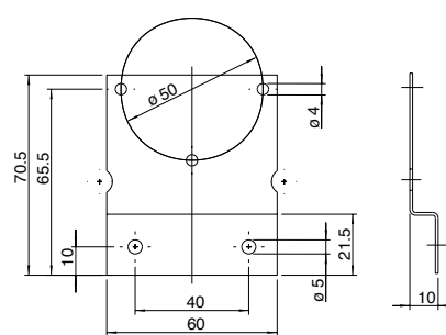
Монтажный уголок 6402
