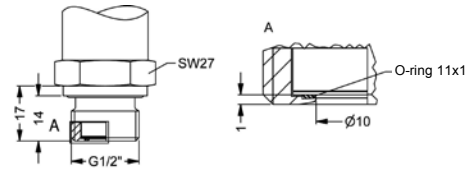
G1/2" semi-flush DIN 3852; M20x1.5 9
