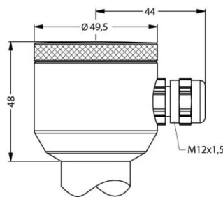
Kompakt-Feldgehäuse (IP 67)
