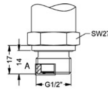
G1/2" quasi-frontbündig DIN 3852; M20x1,5 9
